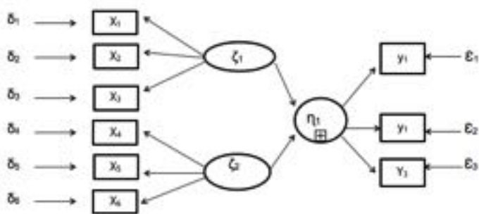
Path diagram d'un model estructural
